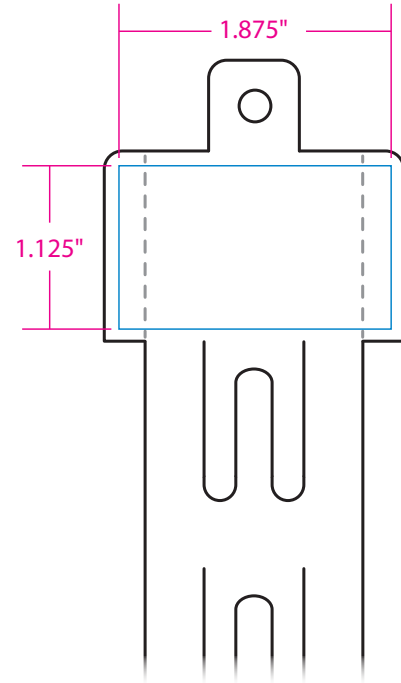
Label Dimensions
