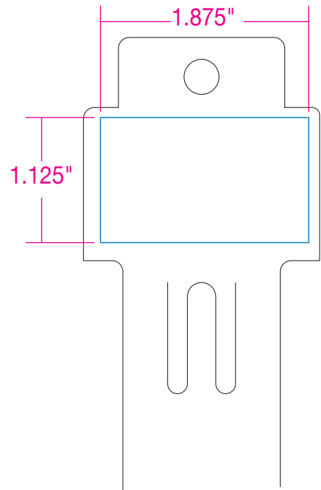
Label Dimensions
